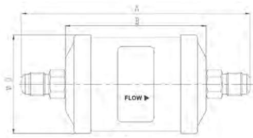
Conexão Rosca
